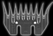
94.5 MM X LONG BEVEL
